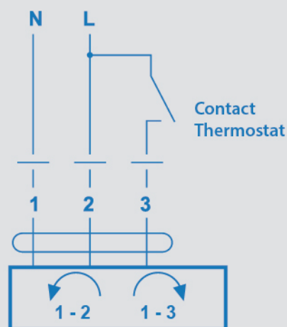
Schéma de câblage du M 24 F-L
