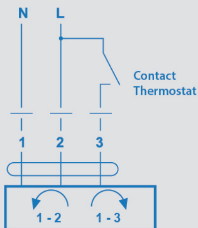
Schéma de câblage du M230 F-L
